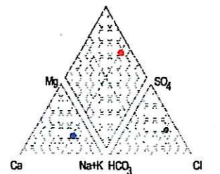
Diagrama de Piper tipo
